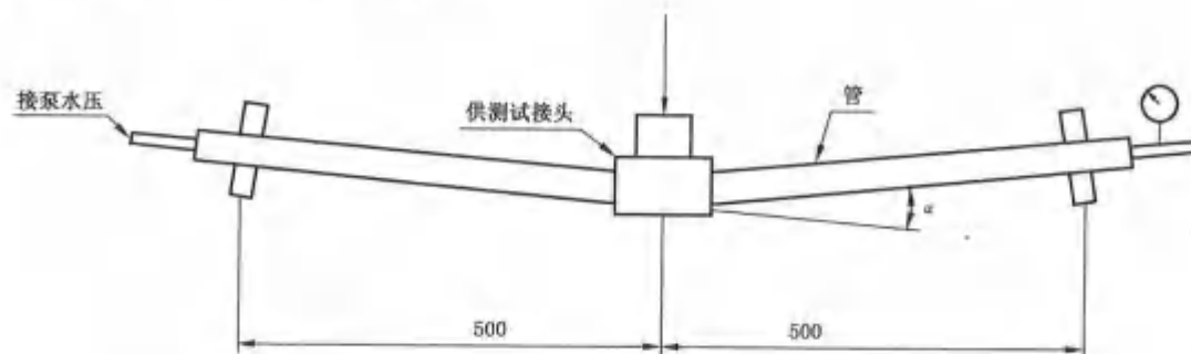
图 13 水压弯曲挠角试验装置
