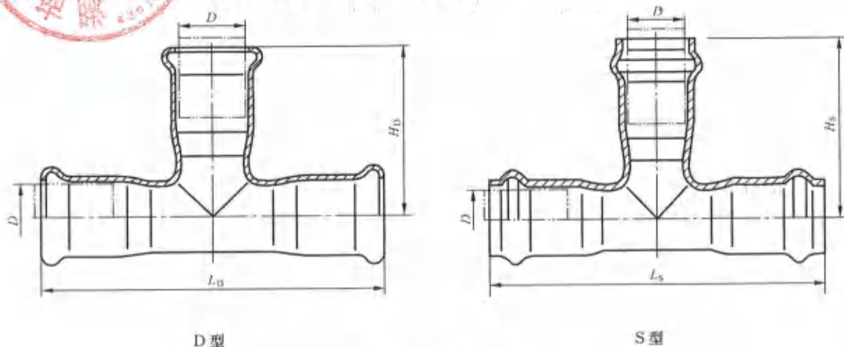
图 5 等径三通
