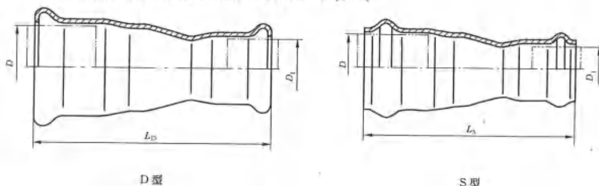
图4 异径接头
