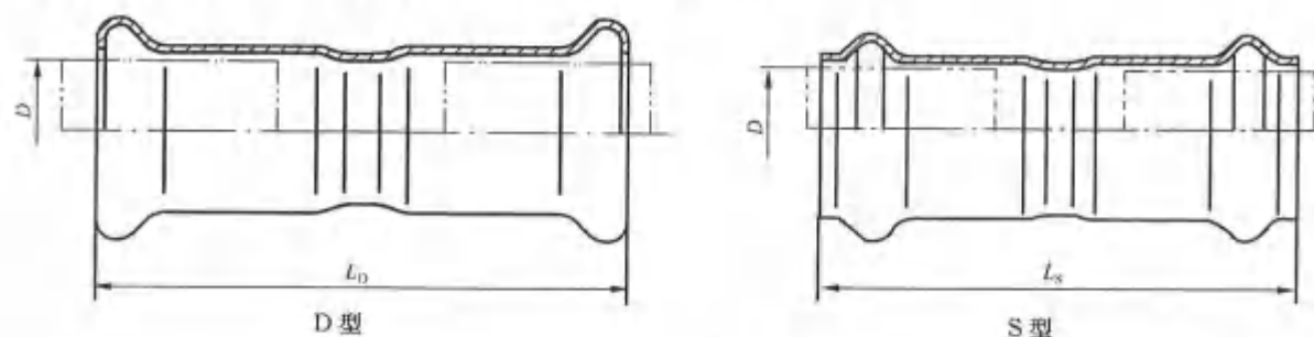
图3 等径接头
