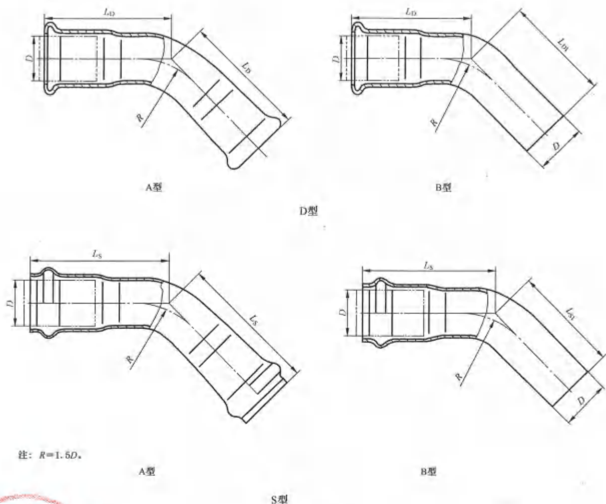
图 8 45°弯头
