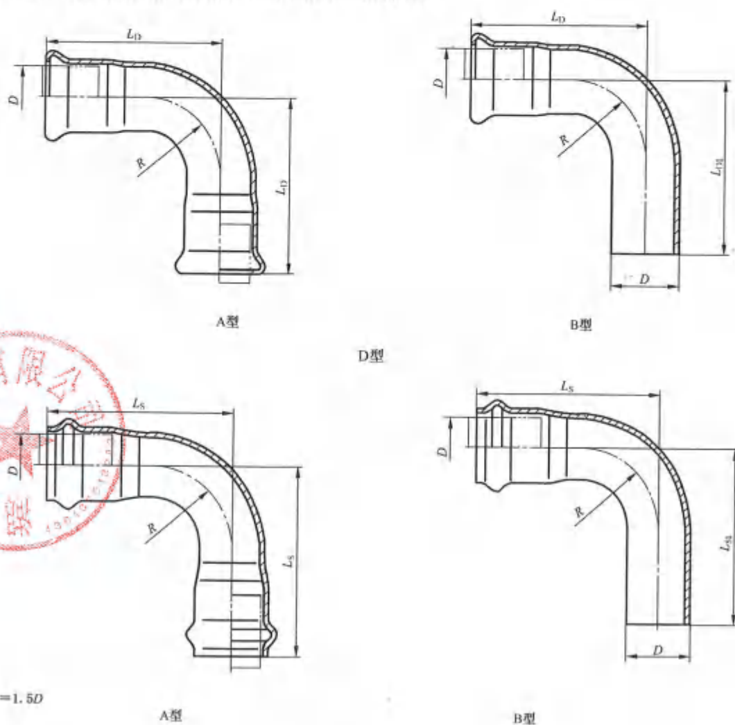
图 7 90°弯头
