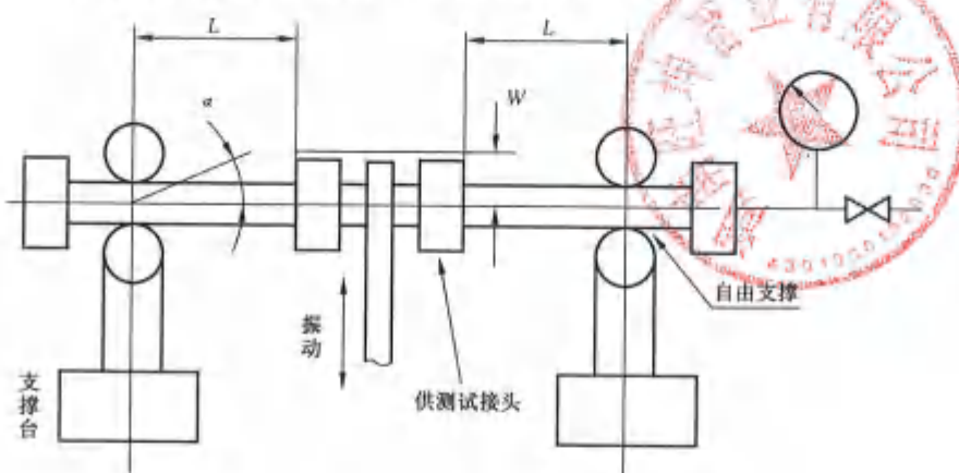
图 14 振动试验装置
