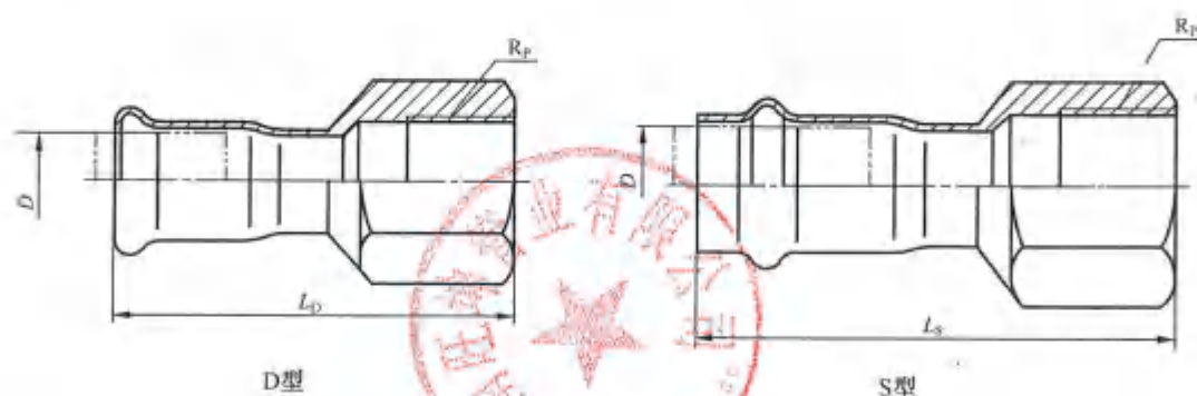
图 9 内螺纹转换接头
