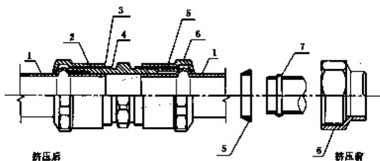
a) 锁紧螺母连接
