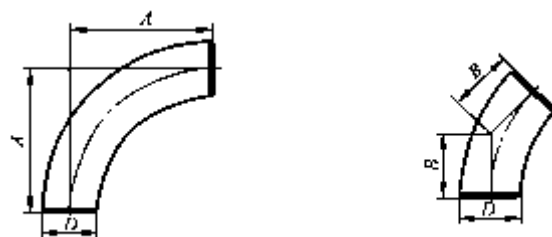
图 6 90°和 45°3D 弯头
