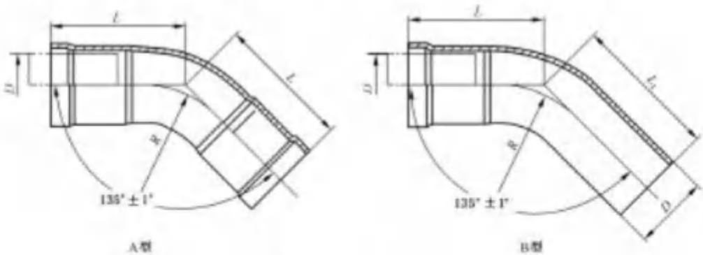
图 A.7 45°弯头
