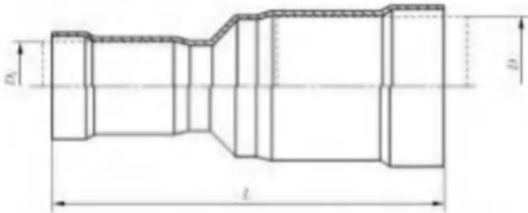
图 A.3 异径接头
