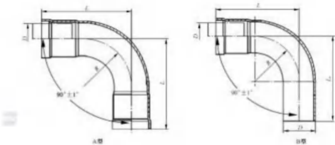
图 A.6 90°弯头
